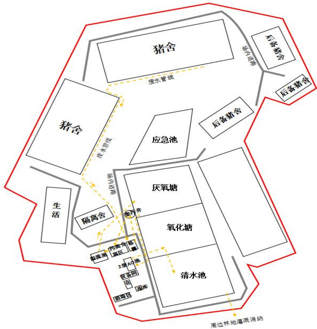
附图3 项目总平面布置图
